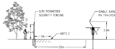
DETAIL 1: TYPICAL ASSET PROTECTION ZONE SECTION SCALE: N.T.S.
